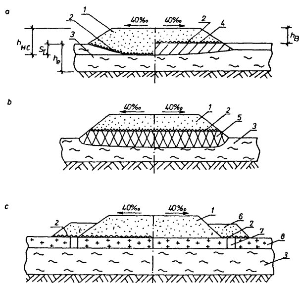
Rys. 3.1. Konstrukcje dróg tymczasowych na gruntach słabonośnych
